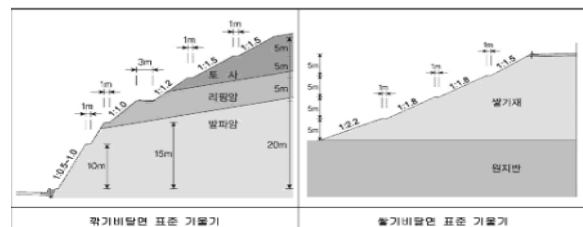
광각비탈면 표준 기울기
