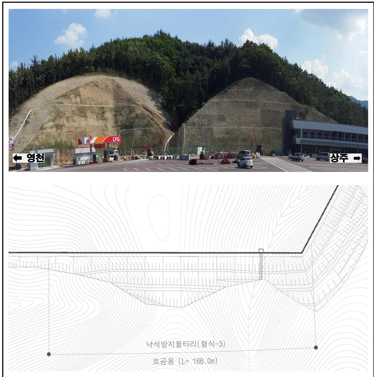
【그림 41.14】 영천절토41 검토대상 비탈면구간
