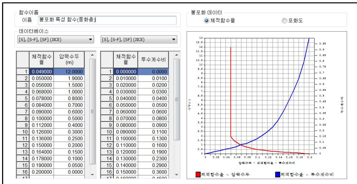
【그림 41.15】 압력수두-체적함수율(포화도)-투수계수비 함수
